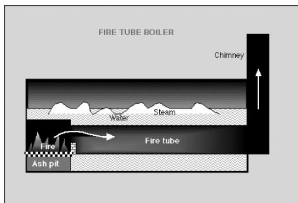
Gambar: Penampang dari boiler tabung api Referensi: http://www.bathtram.org/tfb/tT111.htm
