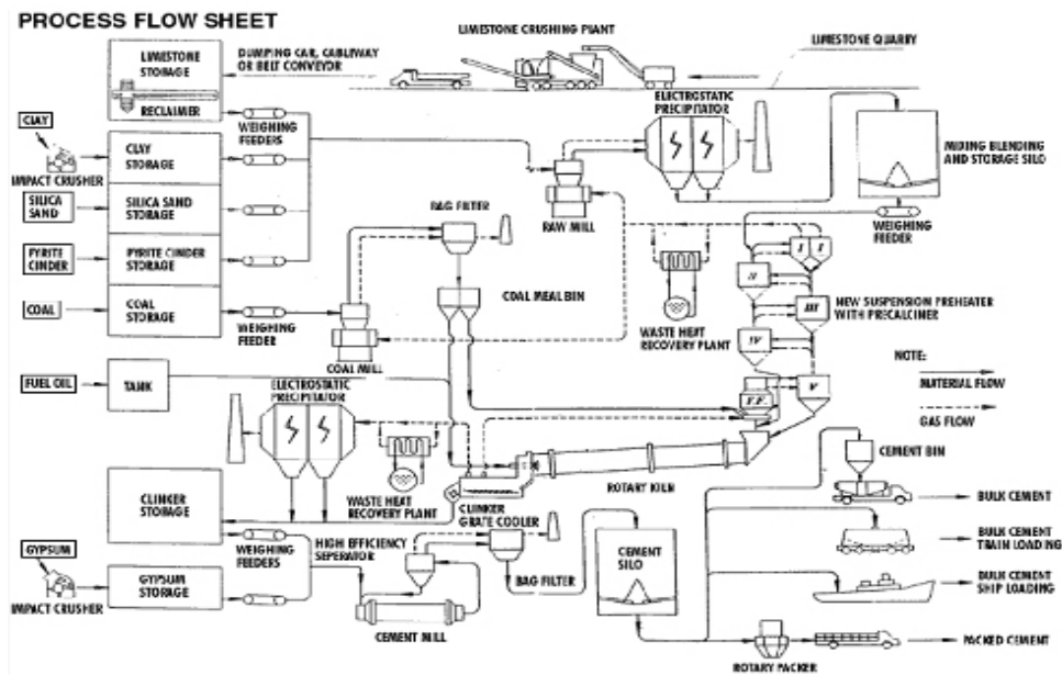
Gambar 1: Proses Produksi Semen. Referensi: http://www.acclimited.com
